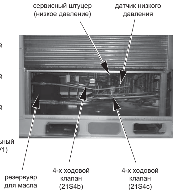
Вид сзади
